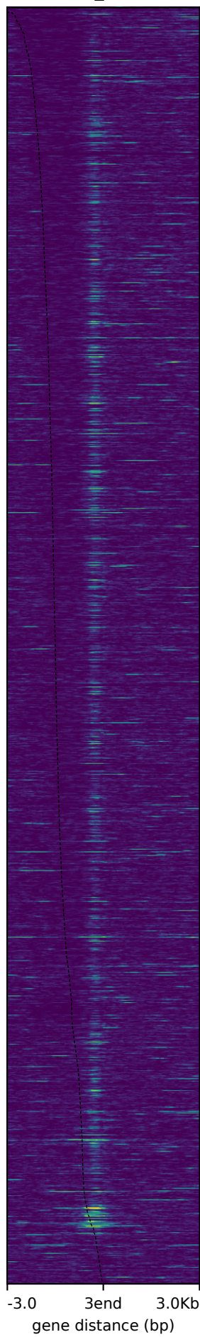
CNCC_NR2F1
